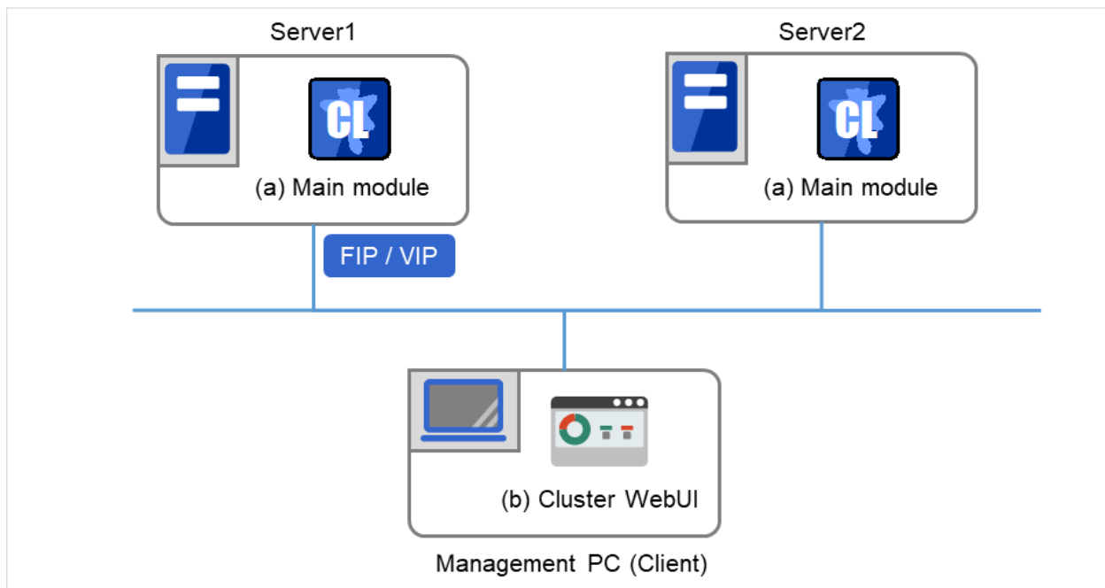
Fig. 6.1: Cluster WebUI
