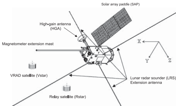
Fig. 1 On-orbit configuration of KAGUYA.
